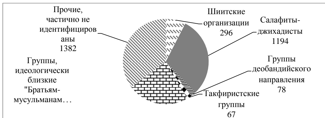
Диаграмма 3. Количество террористических актов в разрезе направленности исламистских организаций за 1968–2009 гг. (подсчитано авторами по базе данных «RAND Database Of Worldwide Terrorism Incidents» 12 )
