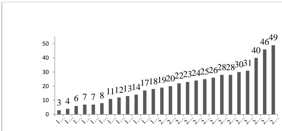
Диаграмма 5. Количество активных бойцов салафитско-джихадистских групп (1988–2013 гг.) [9]
