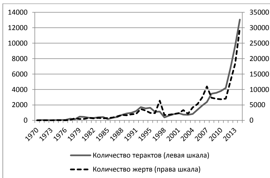
Диаграмма 1. Динамика количества террористических актов, совершенных в странах с преимущественно мусульманским населением, и жертв за 1970–2014 гг. (подсчитано авторами по базе данных «Global Terrorism Data base») 6
