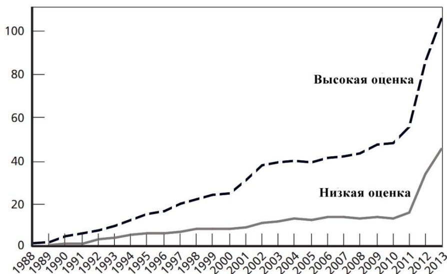
Диаграмма 5. Количество активных бойцов салафитско-джихадистских групп (1988–2013 гг.) [9]
