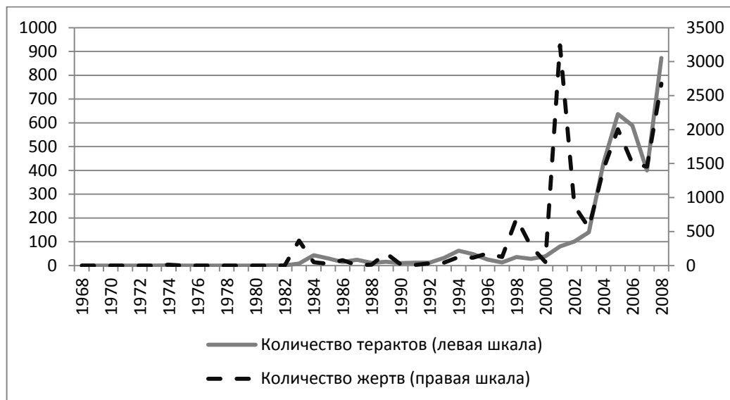
Диаграмма 2. Количество террористических актов, совершенных исламистскими организациями, и жертв подобных терактов за 1968–2008 гг. (подсчитано авторами по базе данных «RAND Database Of Worldwide Terrorism Incidents» 11 )
